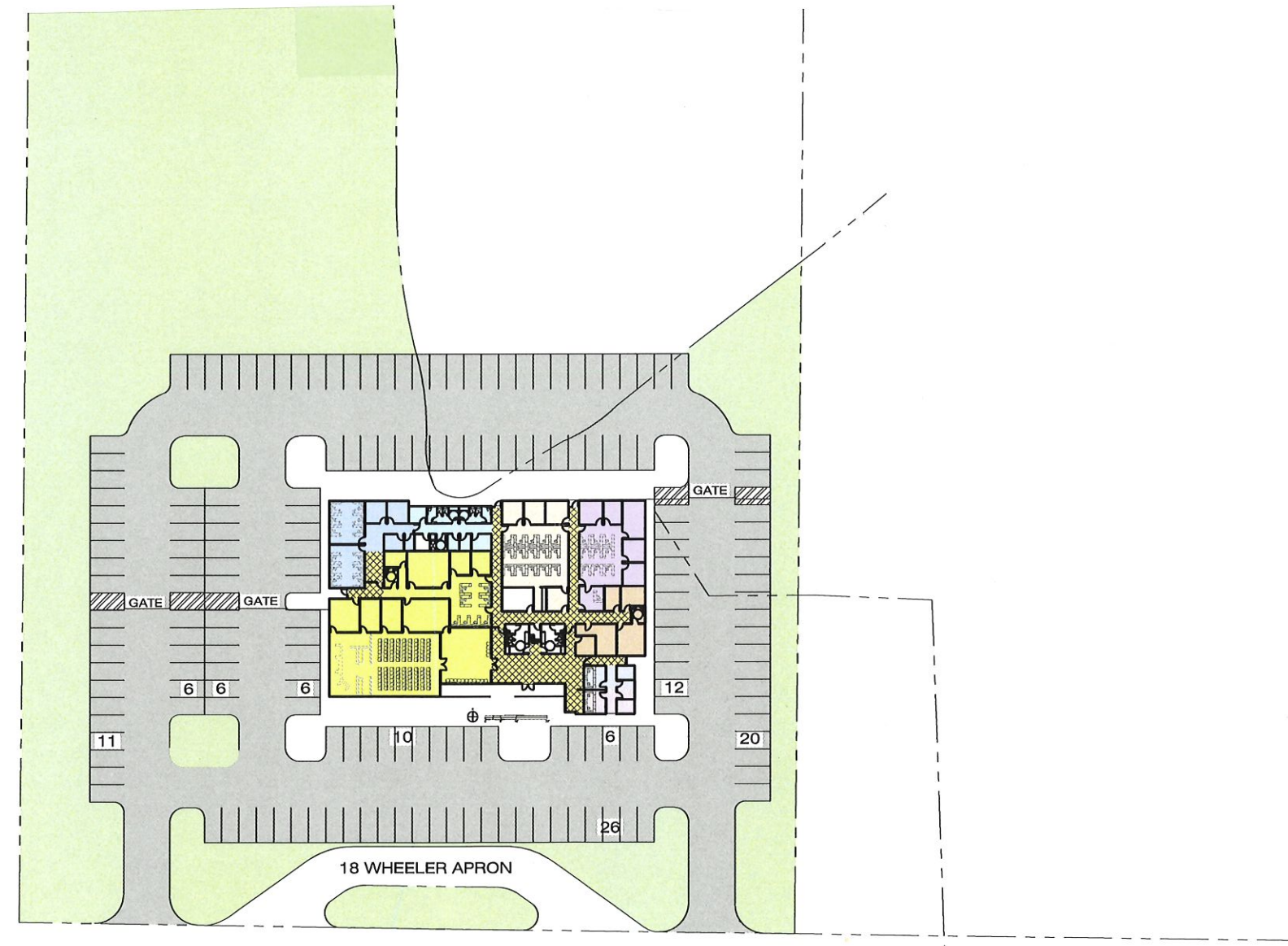
OPTION 2 SITE PLAN
